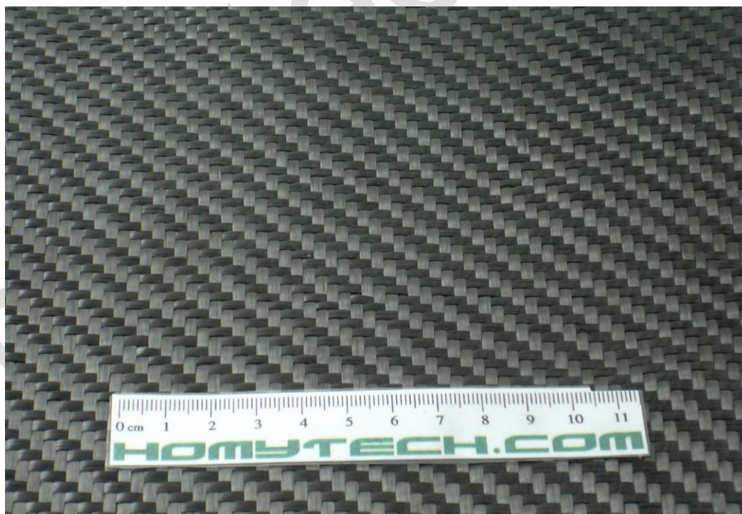
G50-S30-12K 高強度碳纖維紗織成 12K 高強度碳纖維布(斜織)G50-S30B12K 產品照片:
